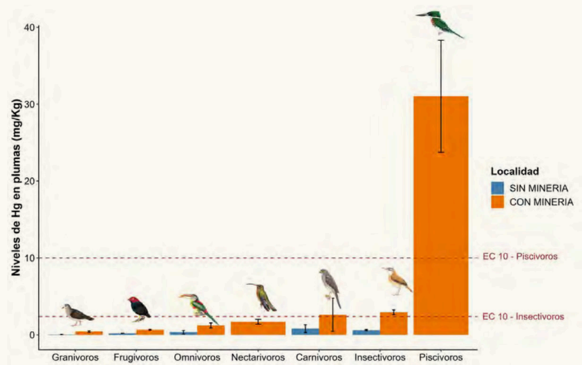
FIGURA 13. CONCENTRACIONES DE MERCURIO EN GREMIOS ALIMENTICIOS – AVES 13
