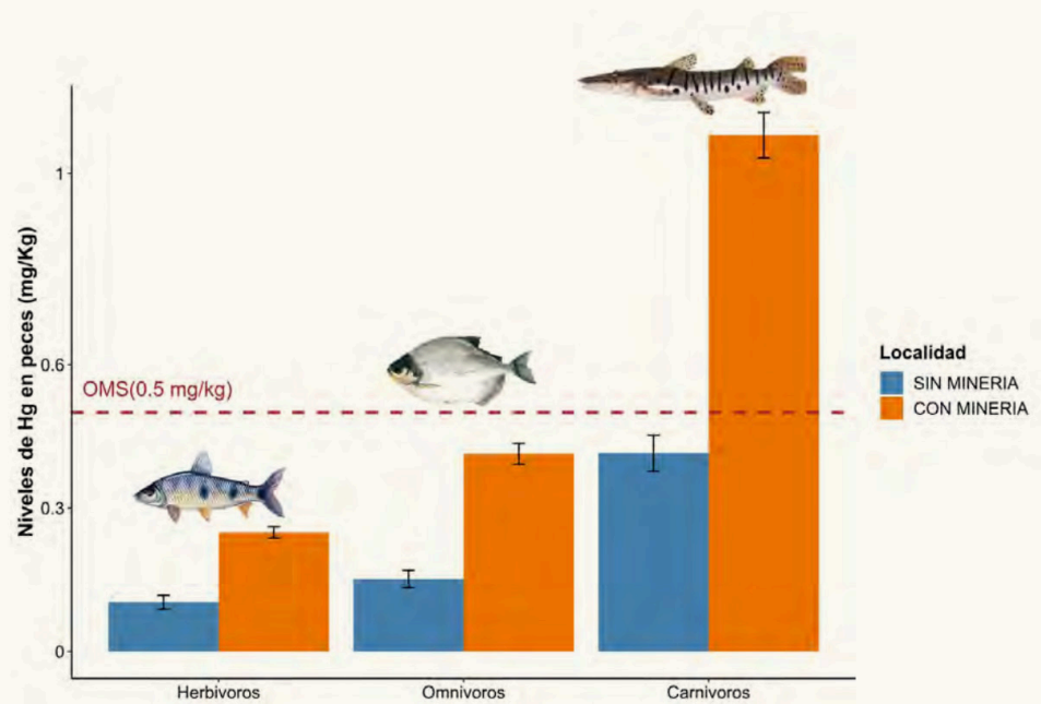
FIGURA 12. CONCENTRACIONES DE MERCURIO EN GREMIOS ALIMENTICIOS – PECES 12
