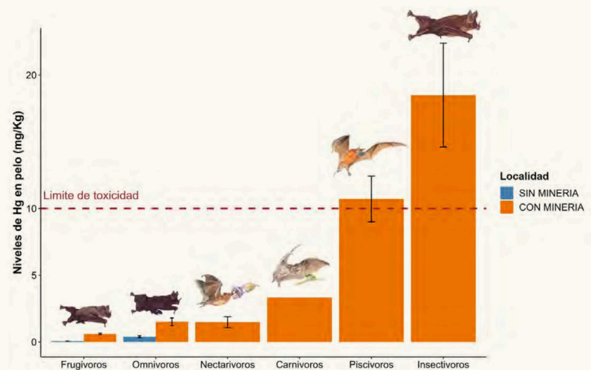
FIGURA 14. CONCENTRACIONES DE MERCURIO EN GREMIOS ALIMENTICIOS – MURCIÉLAGOS 14
